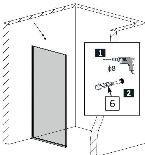
Мал. 35 (вигляд спереду)
