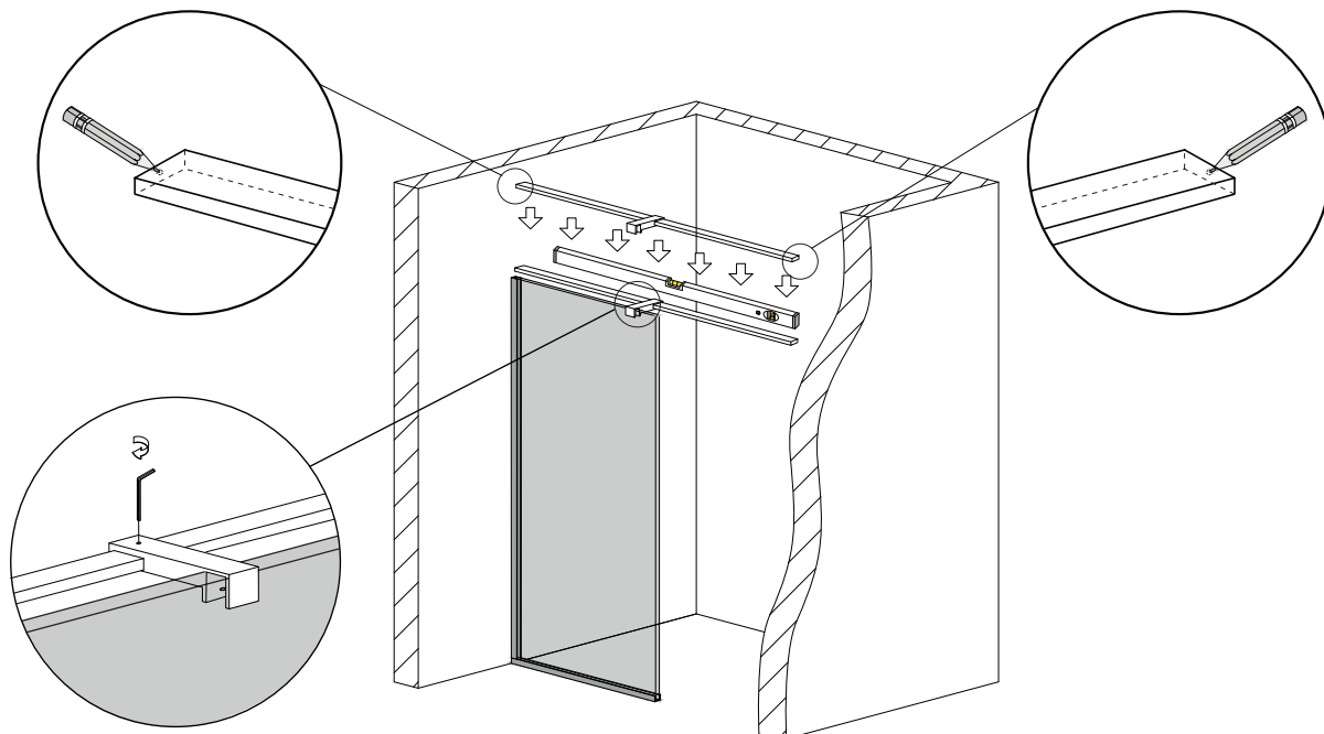
Мал. 25 (вигляд спереду)
