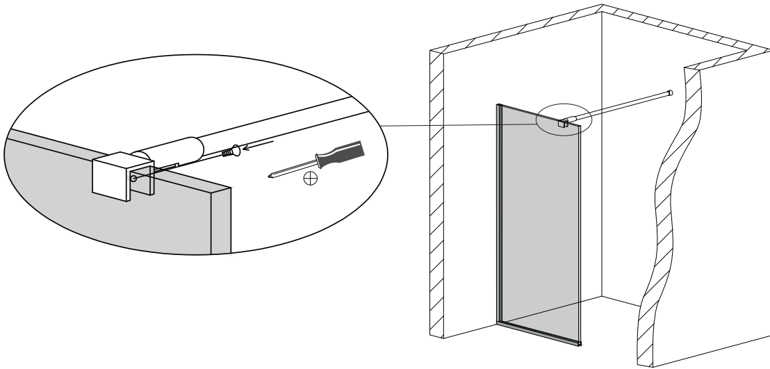
Мал. 42 (вигляд спереду)
