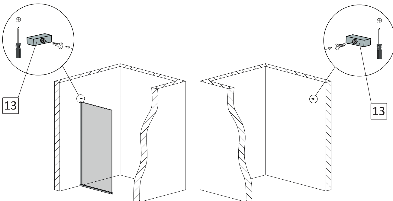
Мал. 28а (вигляд спереду)
