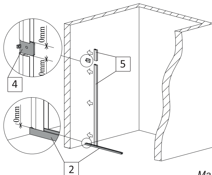
Мал. 9 (вигляд спереду)
