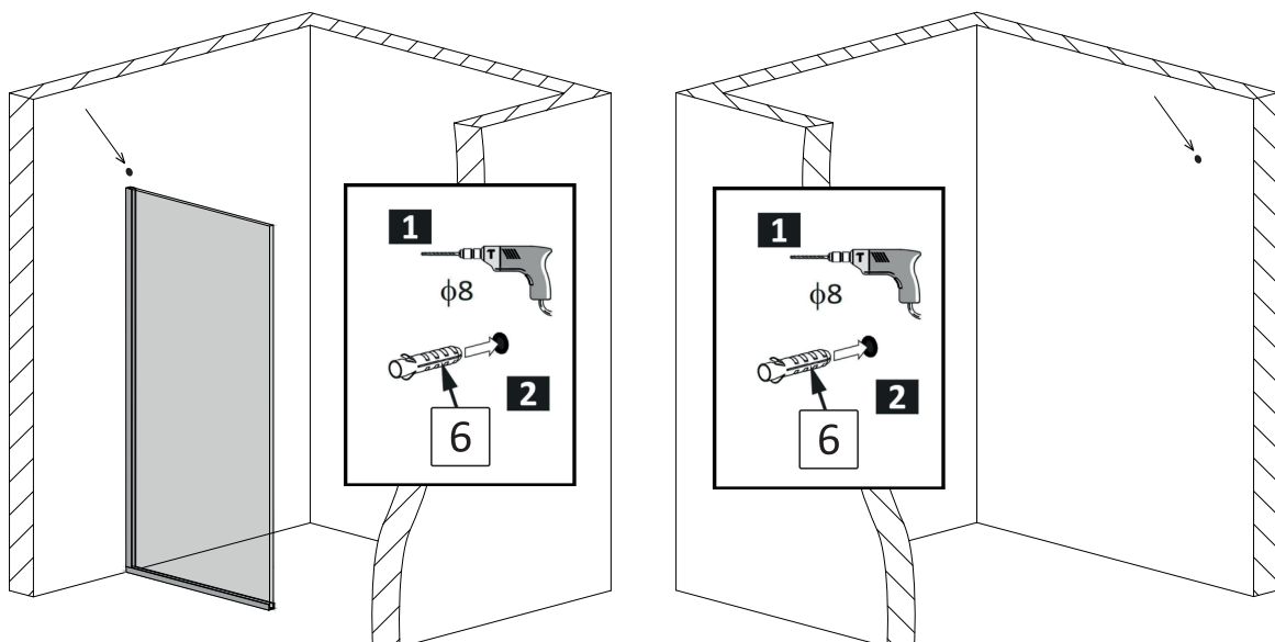
Мал. 21а (вигляд спереду)
