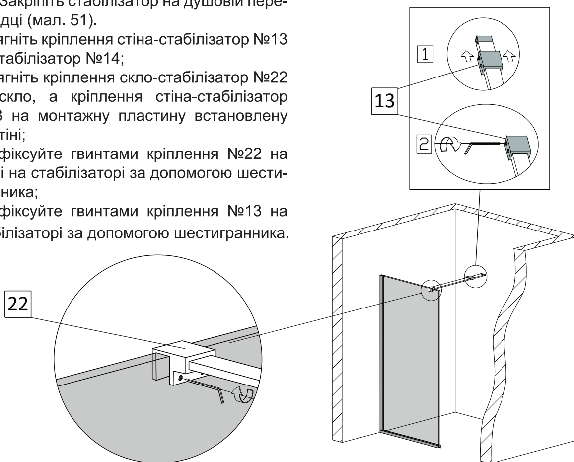
Мал. 51 (вигляд спереду)
